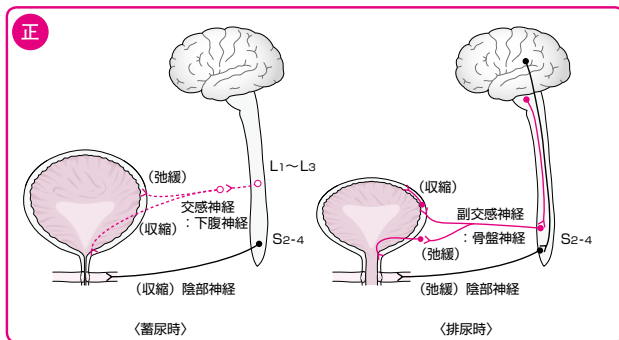
図 7-7 蓄尿と排尿に関わる神経支配
