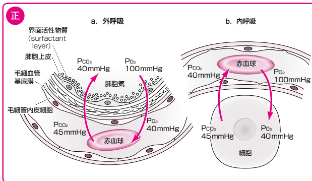
図 6-10 ガス交換のメカニズム
